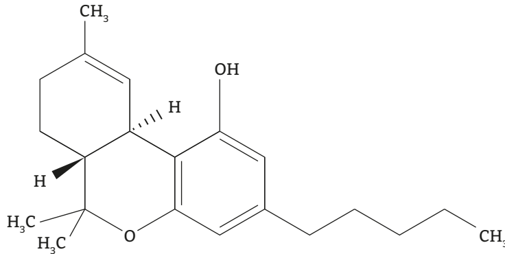
Figura N° 5. Estructura química de \Delta^9 -tetrahydrocannabinol (THC. Fitocannabinoide)
