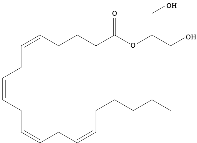
Figura N° 3. Estructura química de 2 AG o 2 araquidonoilglicerol (endocannabinoides)
